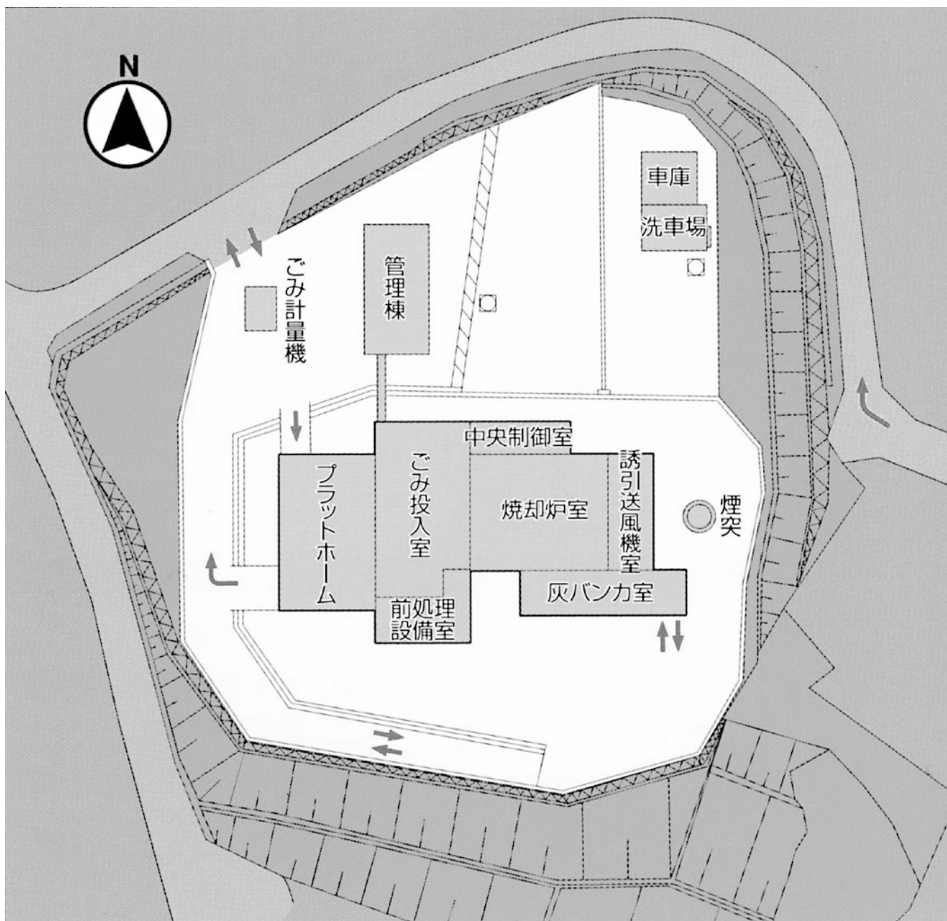
全体配置図
